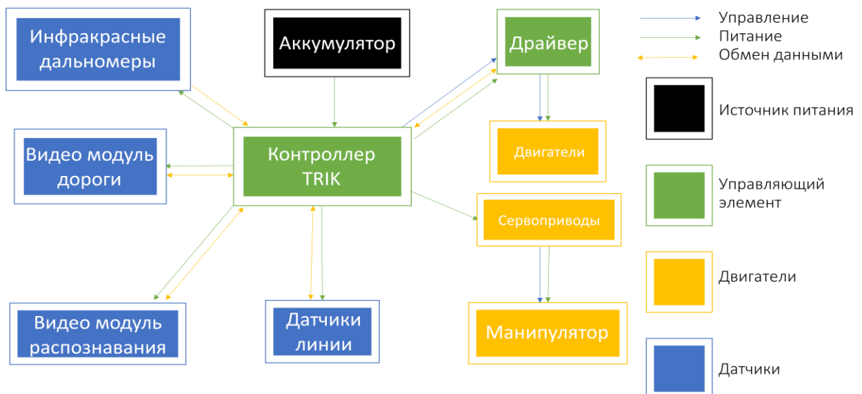
Функциональная схема
