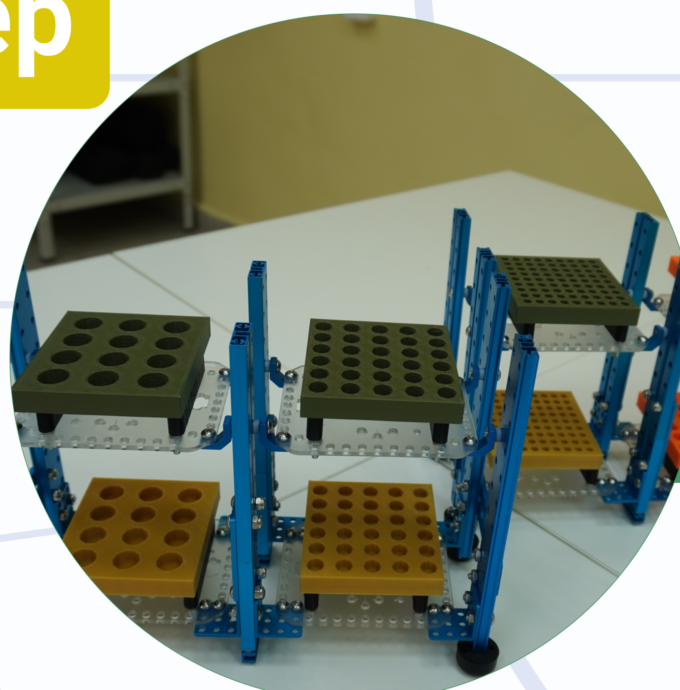
Робот-погрузчик
